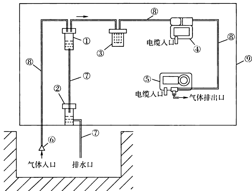
图 1 工艺阀井、地坑及排污沟等场所泵吸式气体采样系统配置示意图
