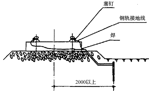
图14 钢轨接地示意（图中尺寸的标注单位为mm）
