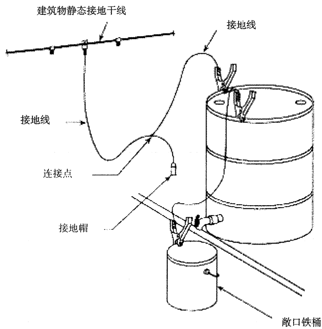
图C.5 分散溶剂设备的典型接地系统连接
