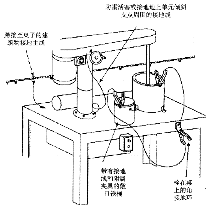
图C.6 小型设备的典型接地系统连接
