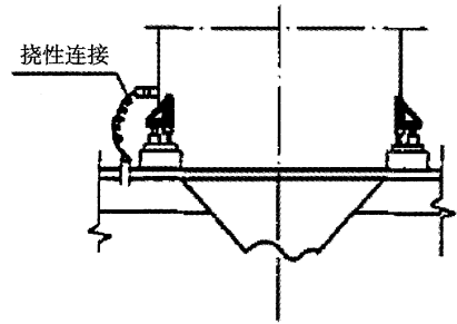
图5 振动设备接地方案
