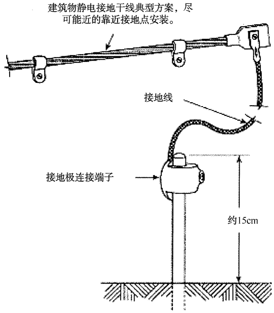
图C.1 接地干线与接地极的连接
