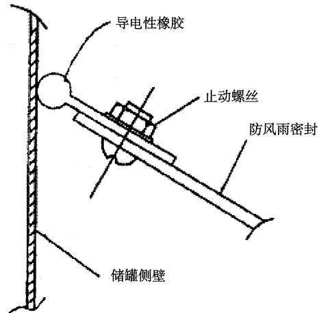
图8 防风雨密封与储罐侧壁的跨接
