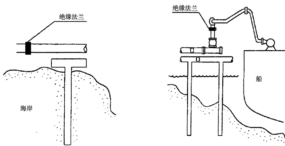
图15 绝缘法兰使用示意
